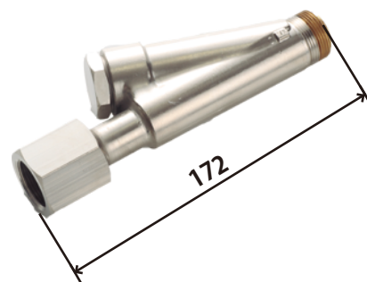
Y型ストレーナ
