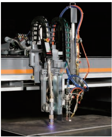
トーチブロック
