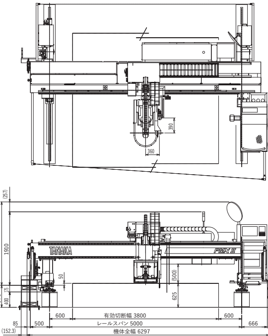
■ KT-790PMX II 機体外観図
