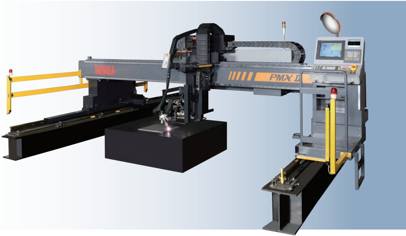
■ KT-790PMX II 機体外観図
