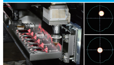
自動ノズルチェンジャシステム
