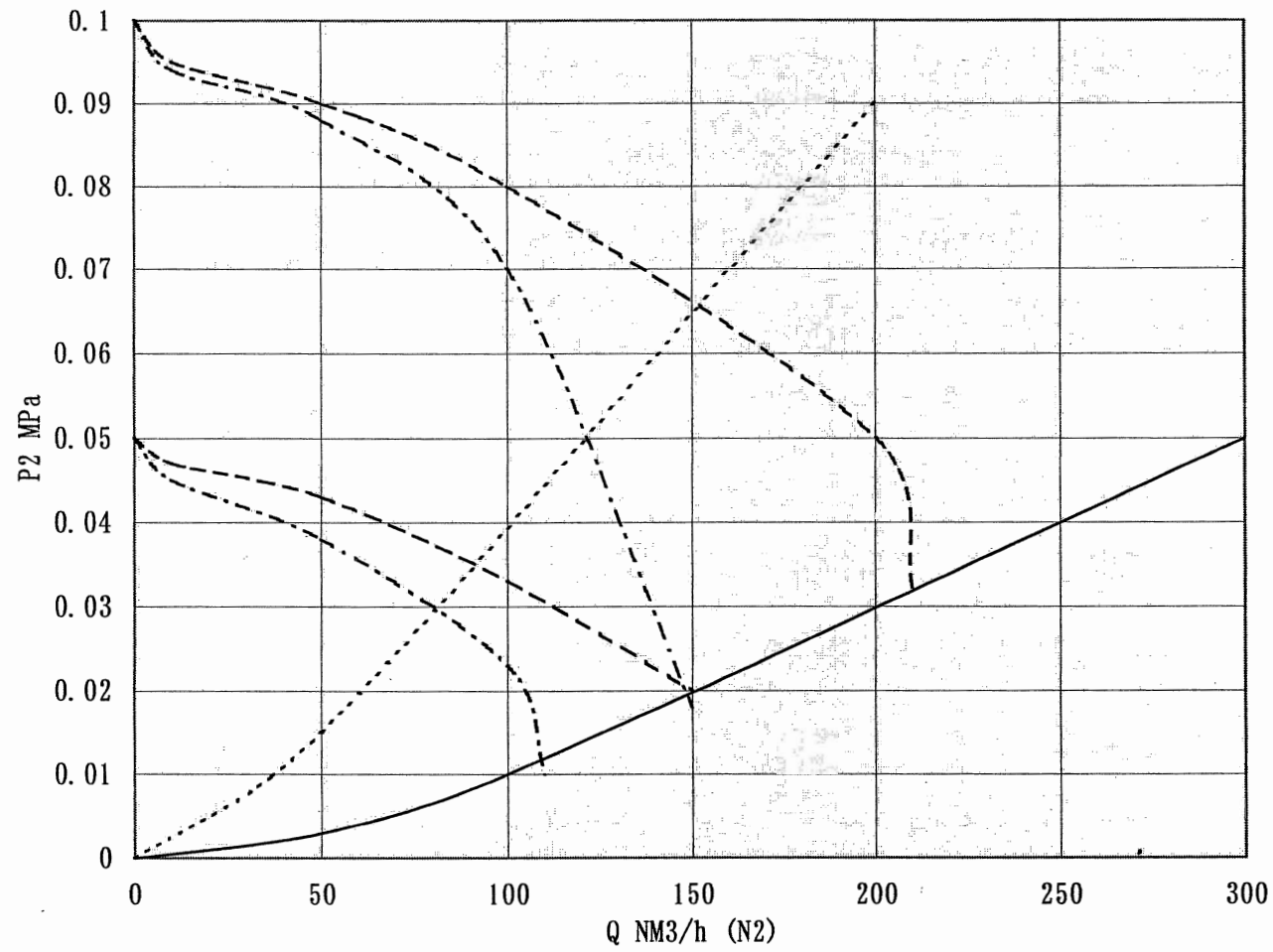
AURORA 3 C2H2, C3H8 P2-Q
