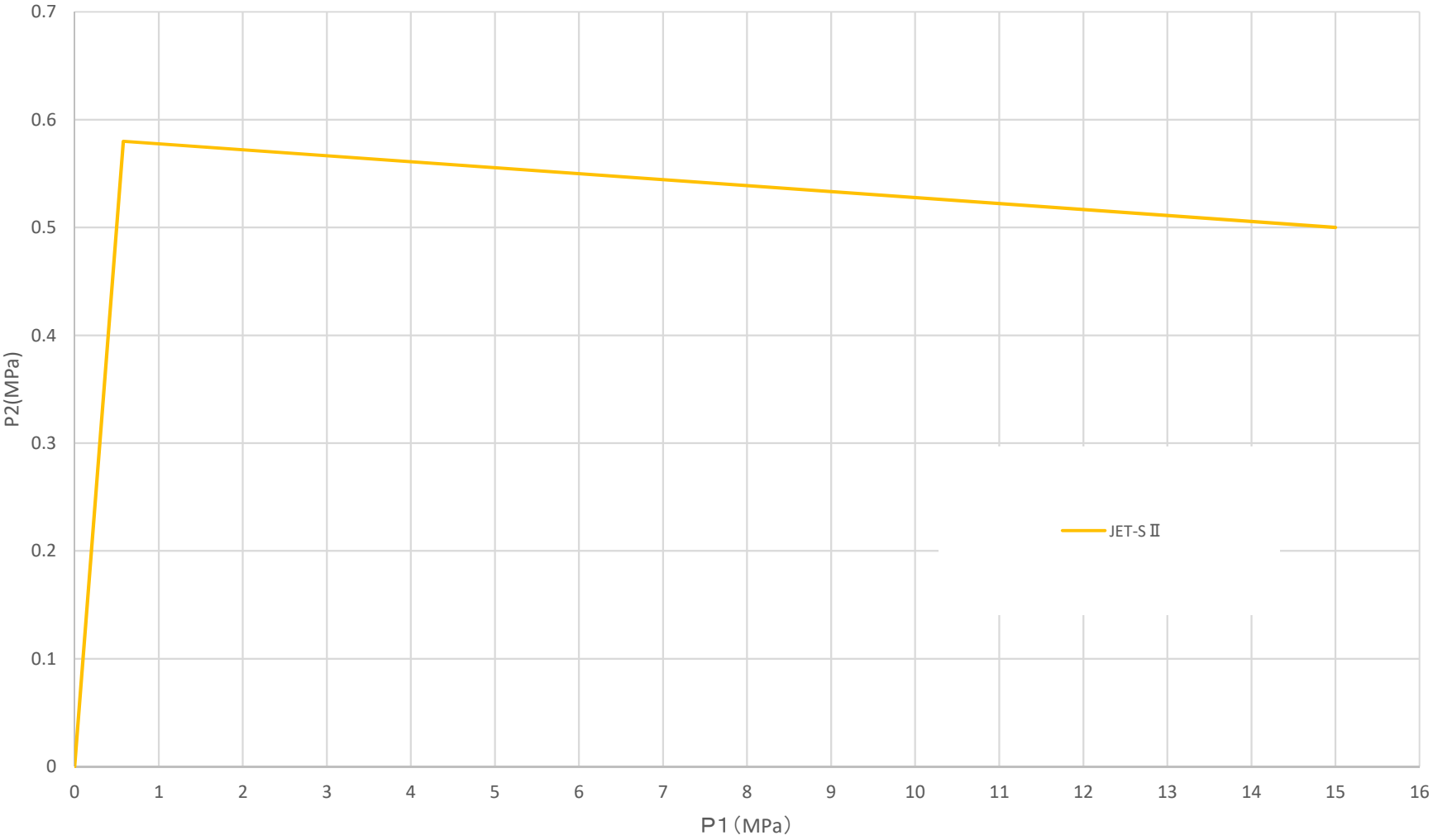
JET-S II P1-P2特性
