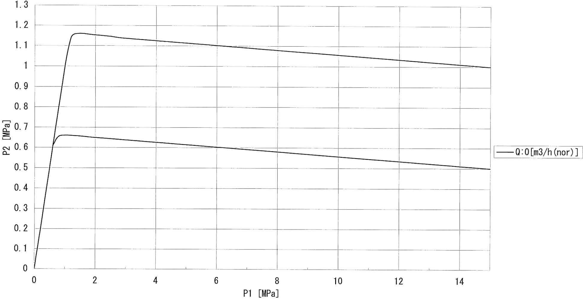
NT50B/NT50S P1-P2特性
