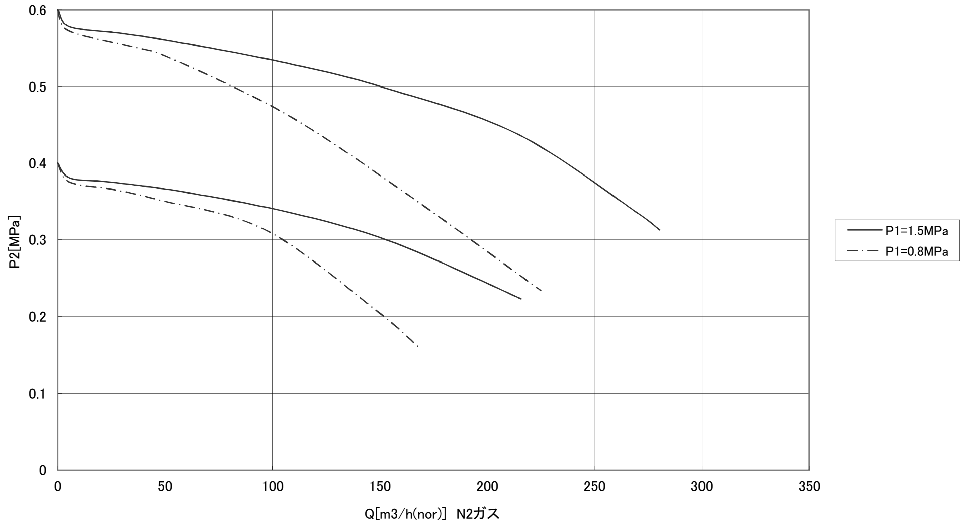
NT100B P2-Q特性
