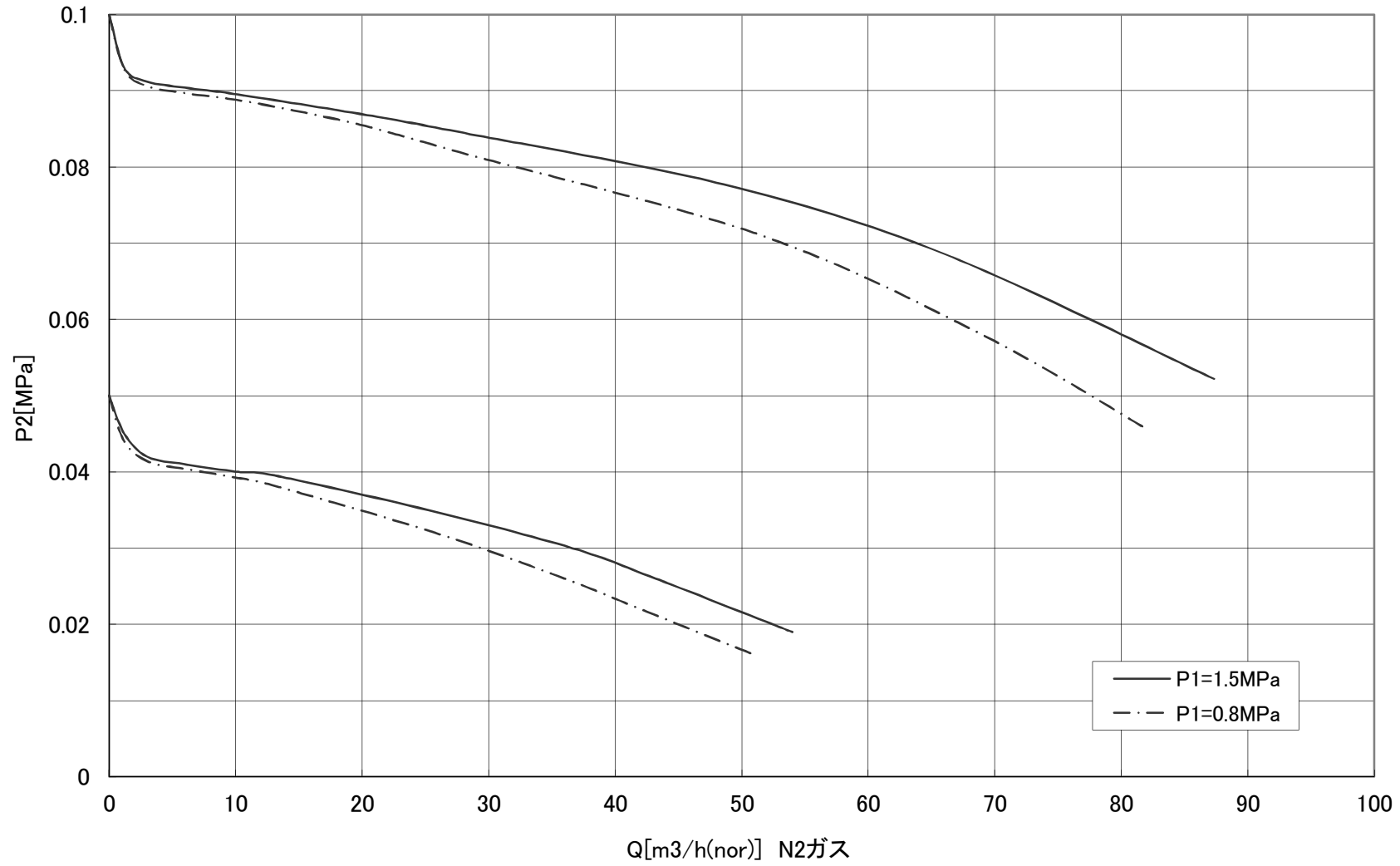
NT100B P2-Q特性
