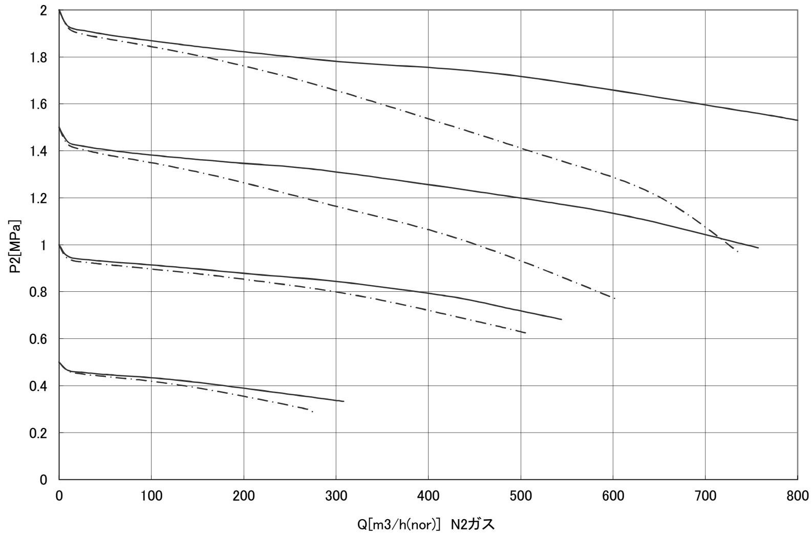
NT100B/NT100S P2-Q特性
