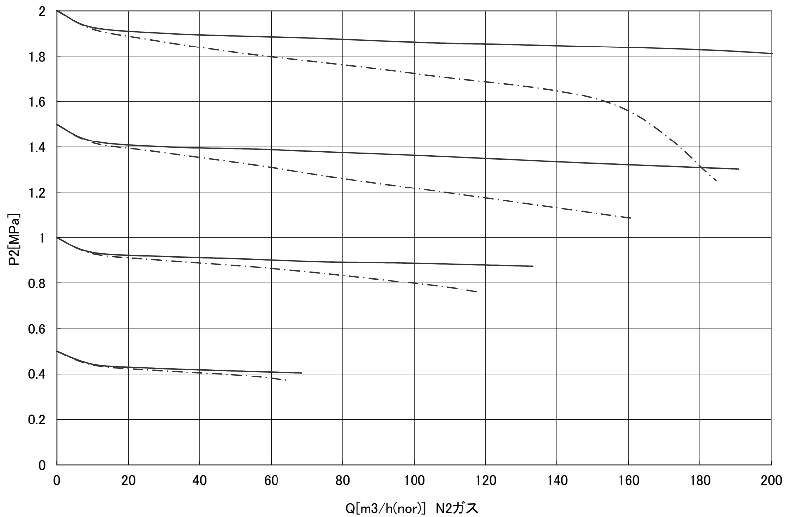
NT50B/NT50S P2-Q特性
