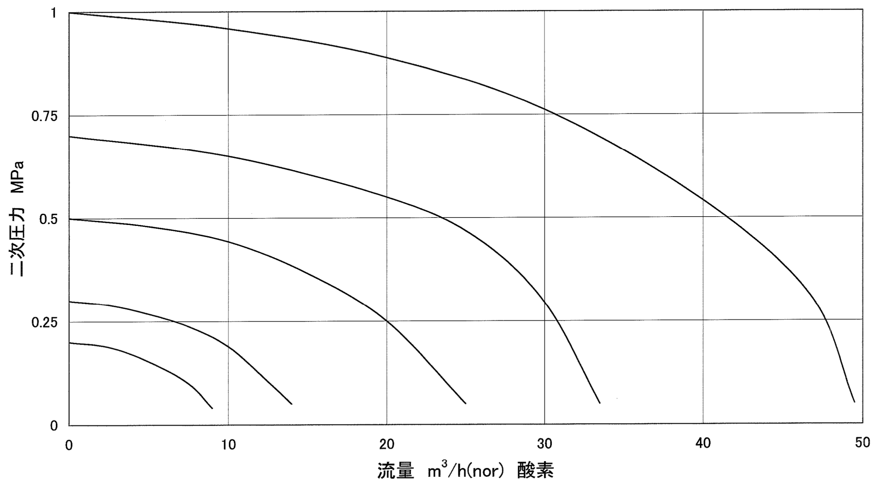
FA-210-O流量特性表
