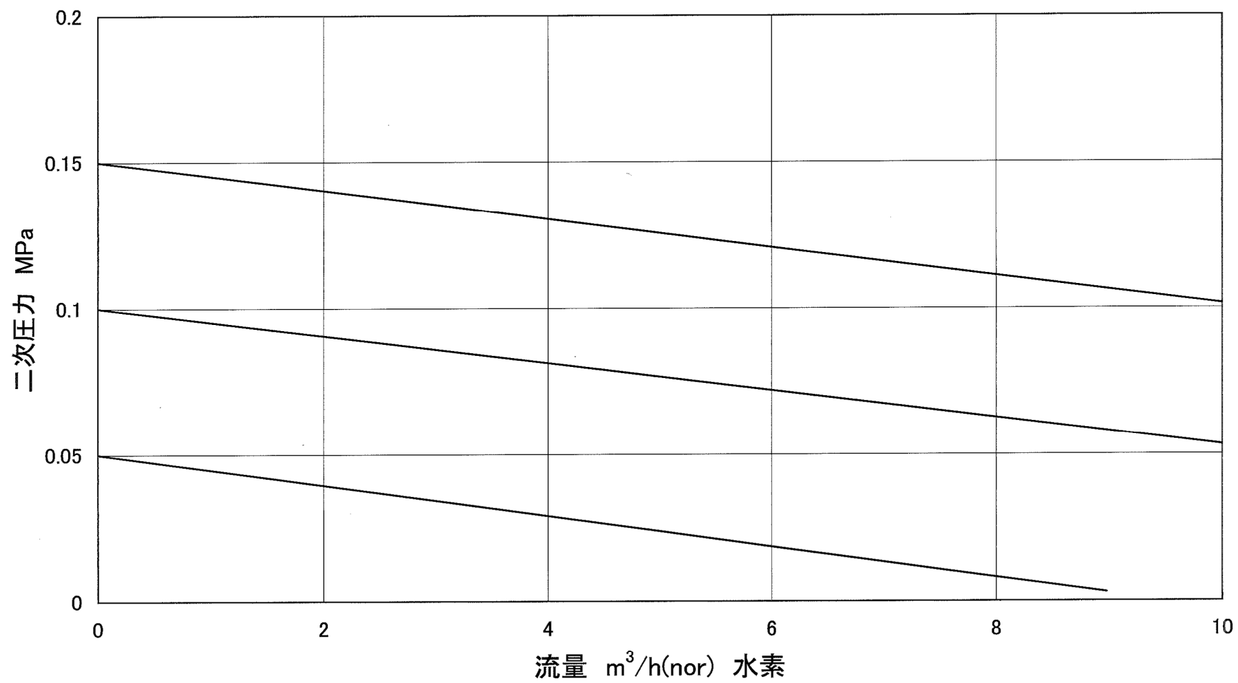
FA-220-H流量特性表
