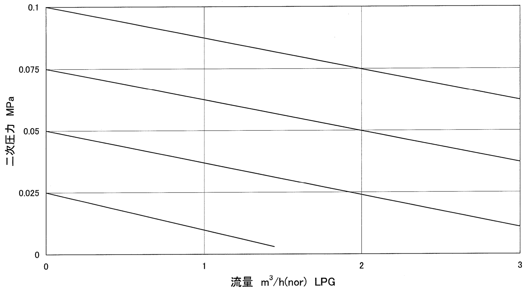
FA-210P流量特性表
