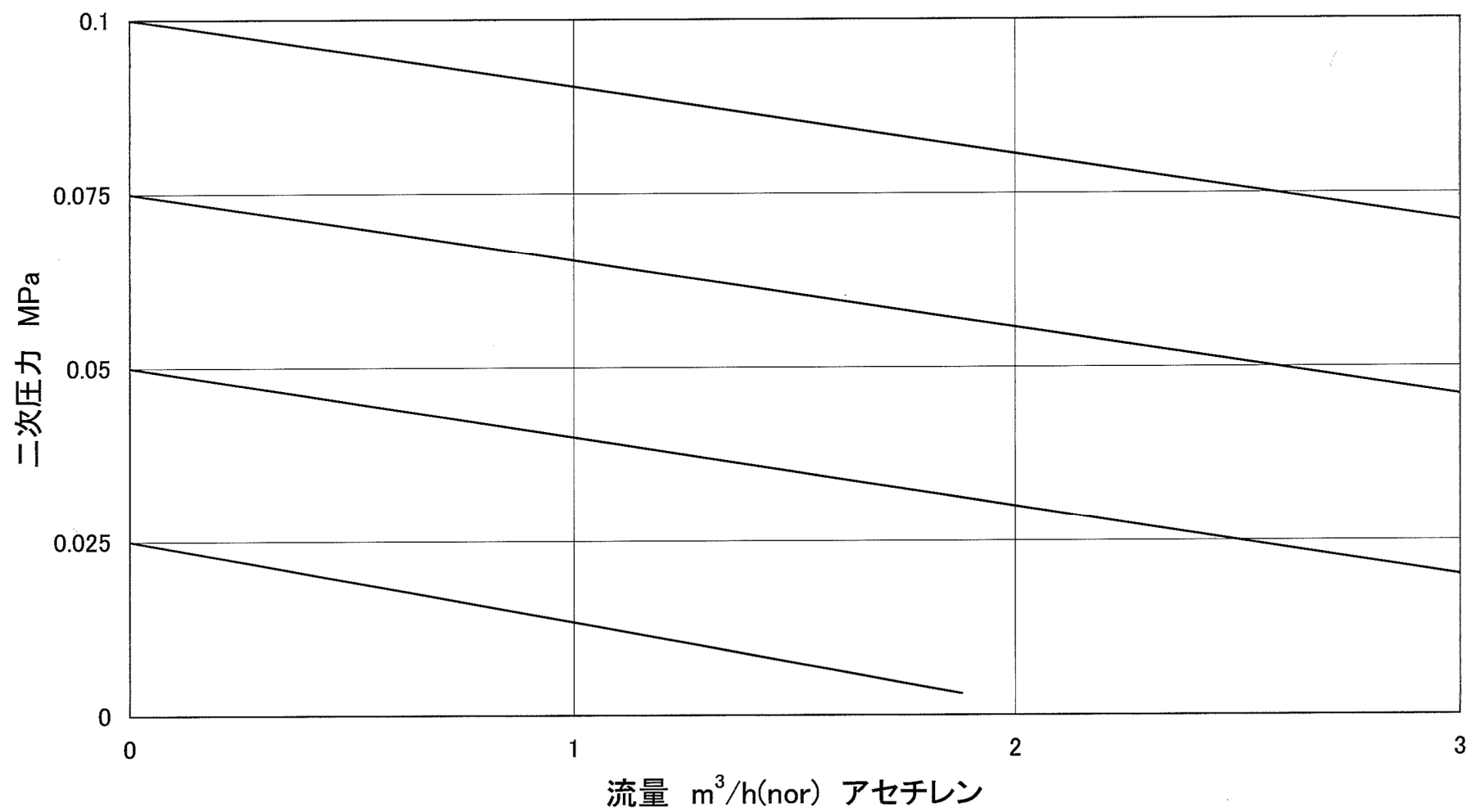
FA-210A流量特性表
