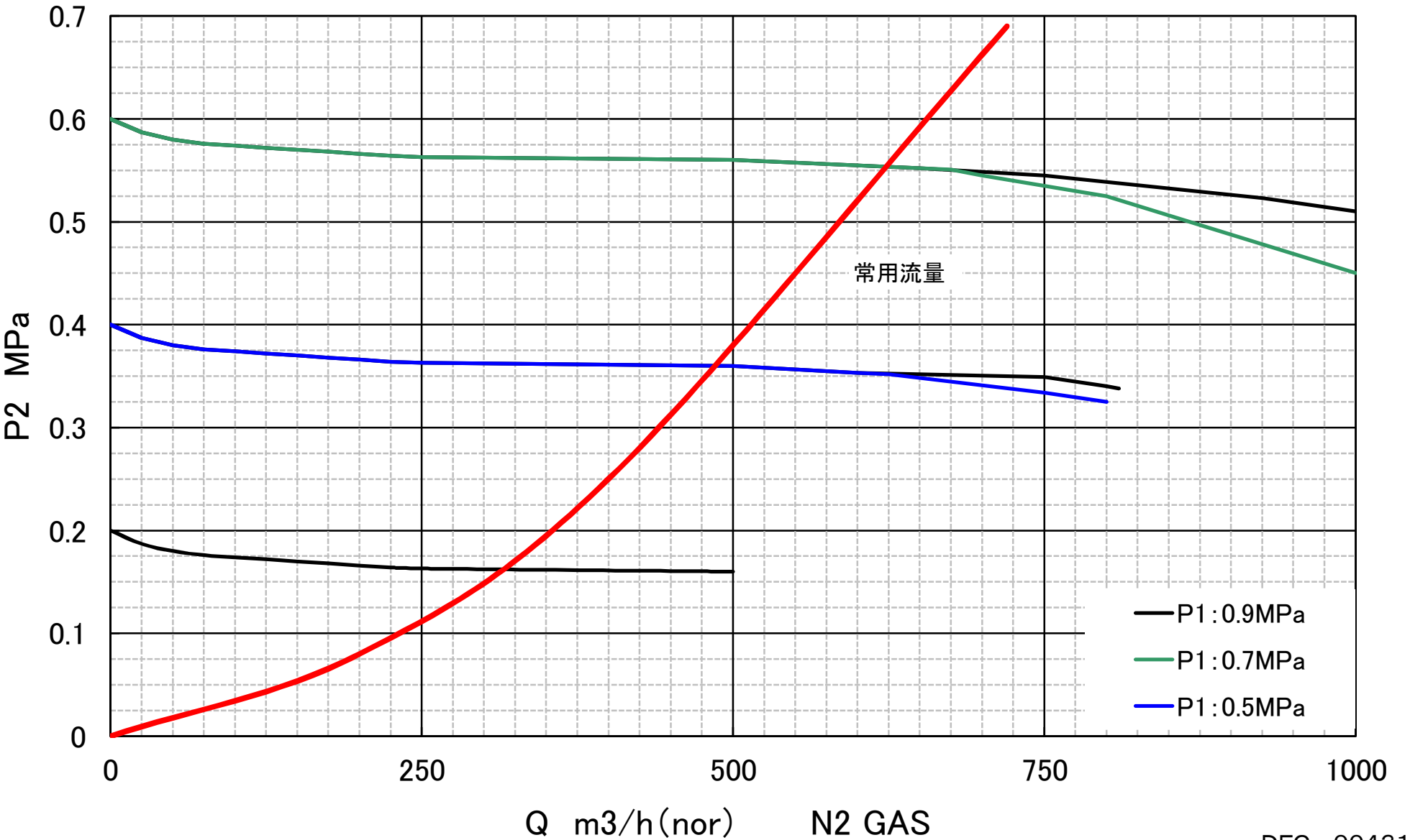
TORR-800Msr P2-Q 特性
