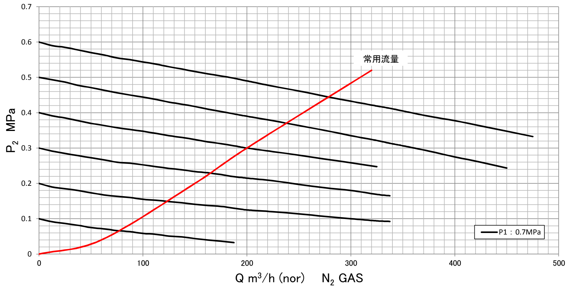
TORR-800G sr P_2 -Q 特性
