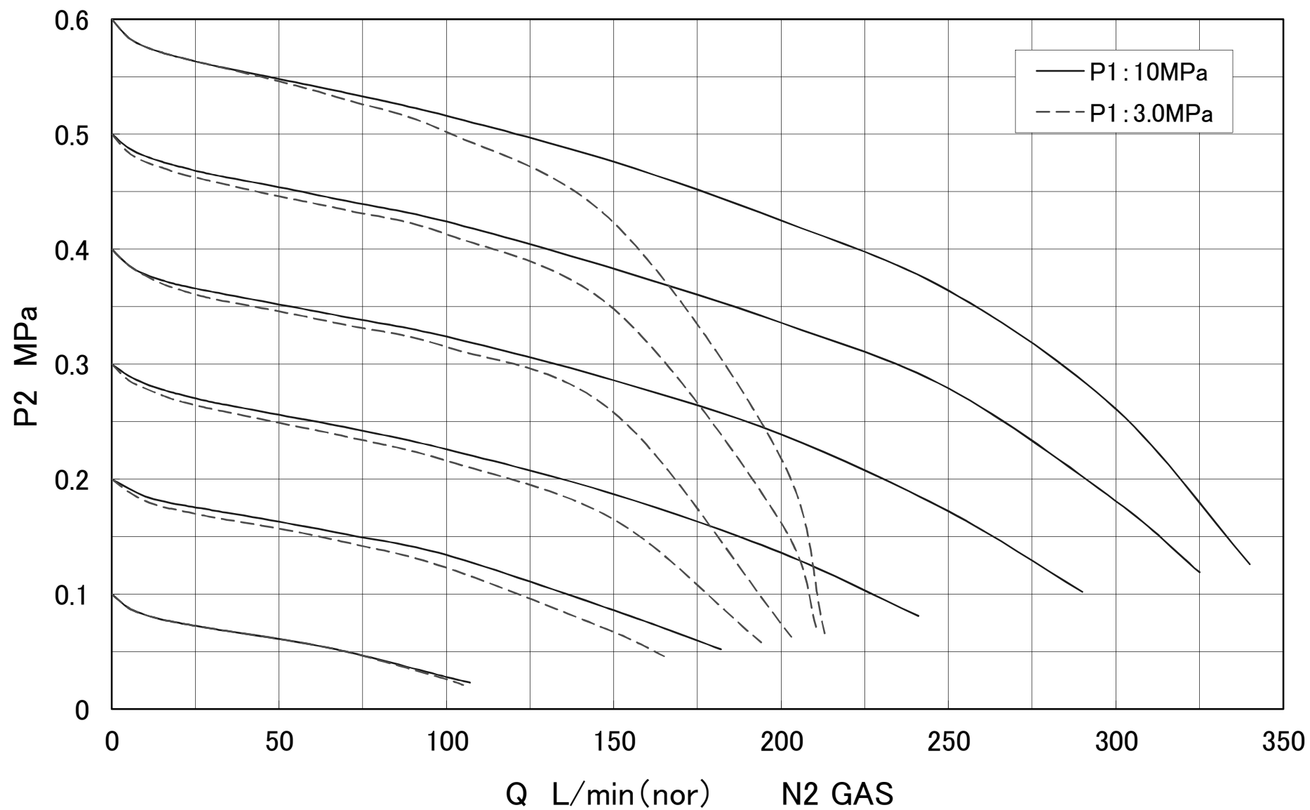
S/LABO B2, S2sr P2-Q 特性
