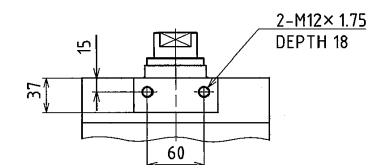
固定用ネジ詳細 (1 / 4)
