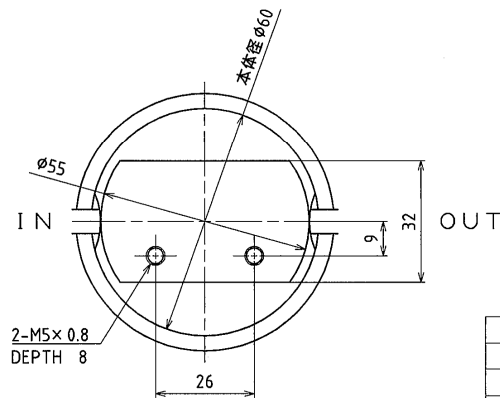
背面図
