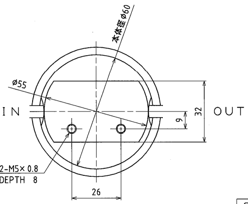
背面図
