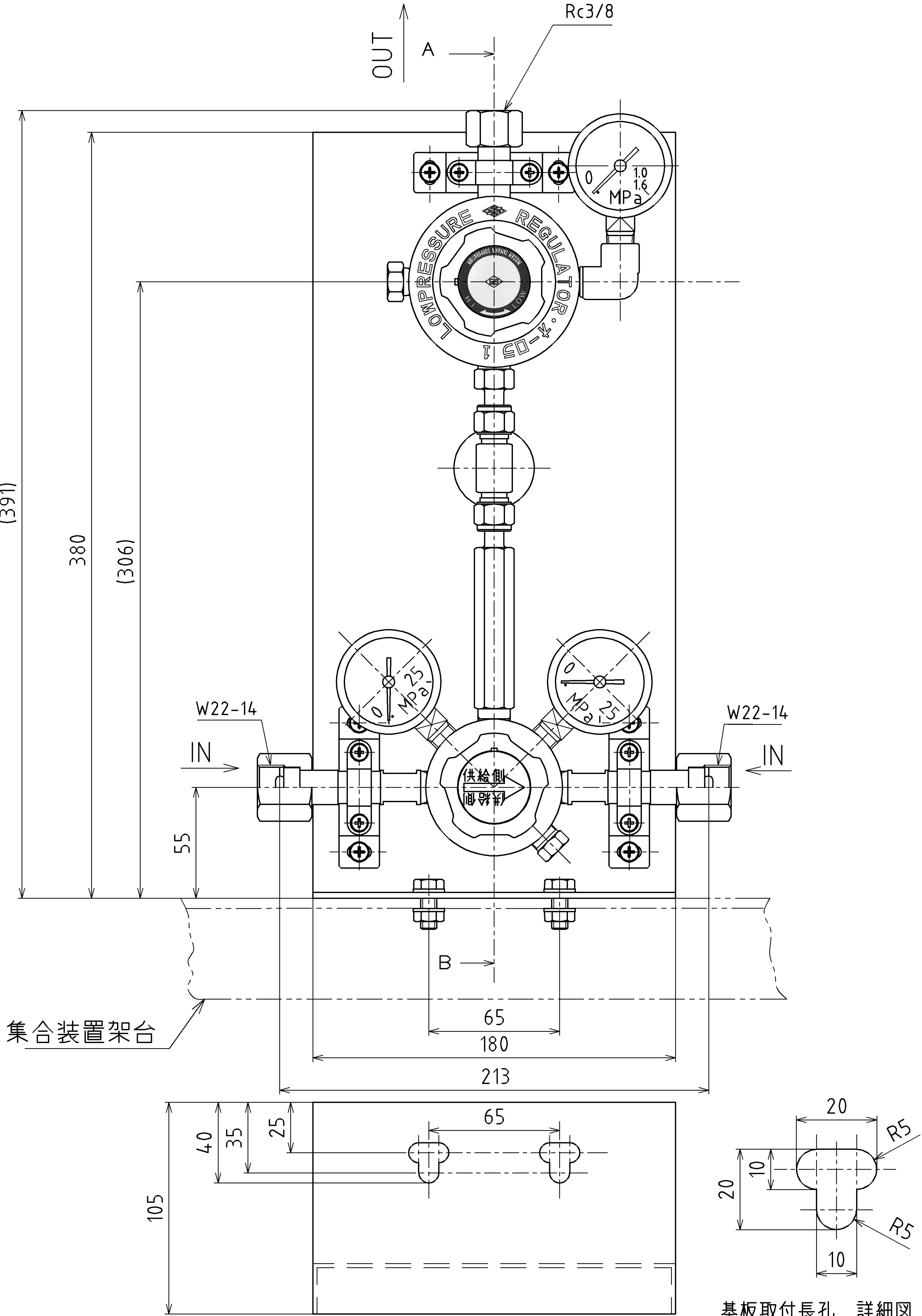
基板取付長孔 詳細図
