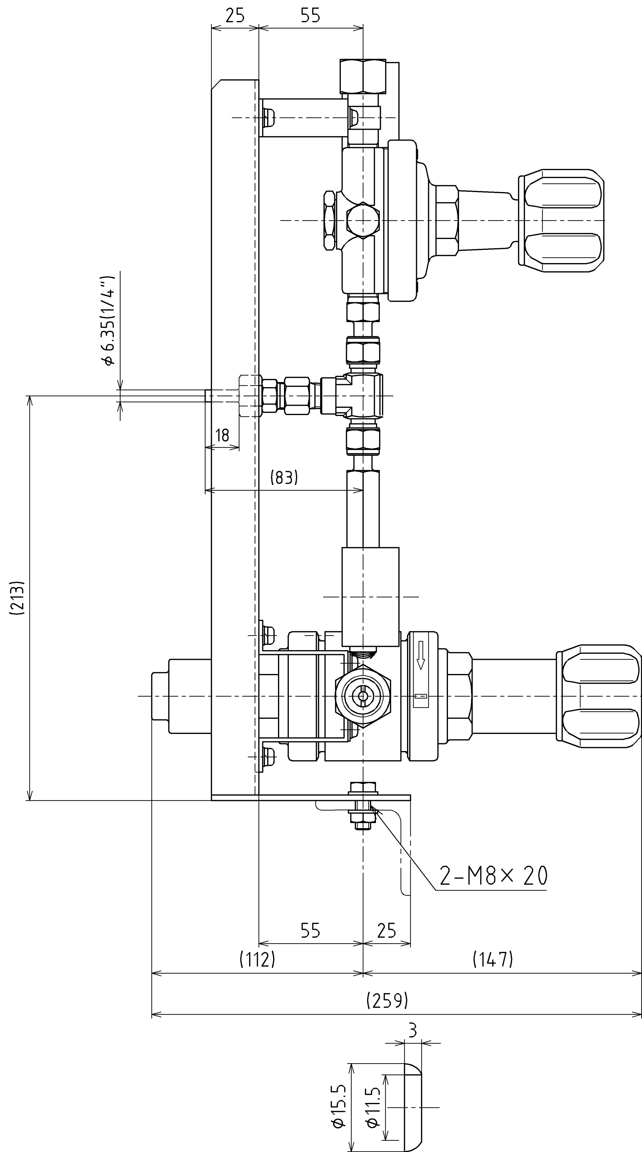
入口メタル当たり用変換リング(付属品) 詳細図
