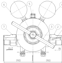
(1) NT100B 出入口接続 W29-16R 当り
