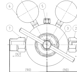
(3) NT100S 出入口接続 W29-16R 当り
