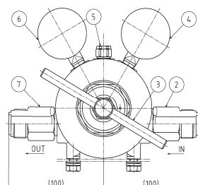
(2) NT100B 出入口接続 W29-16P 当り
